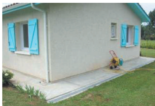
Figure 20 Large trottoir avec caniveau de collecte des eaux de ruissellement (Source Socabat)
